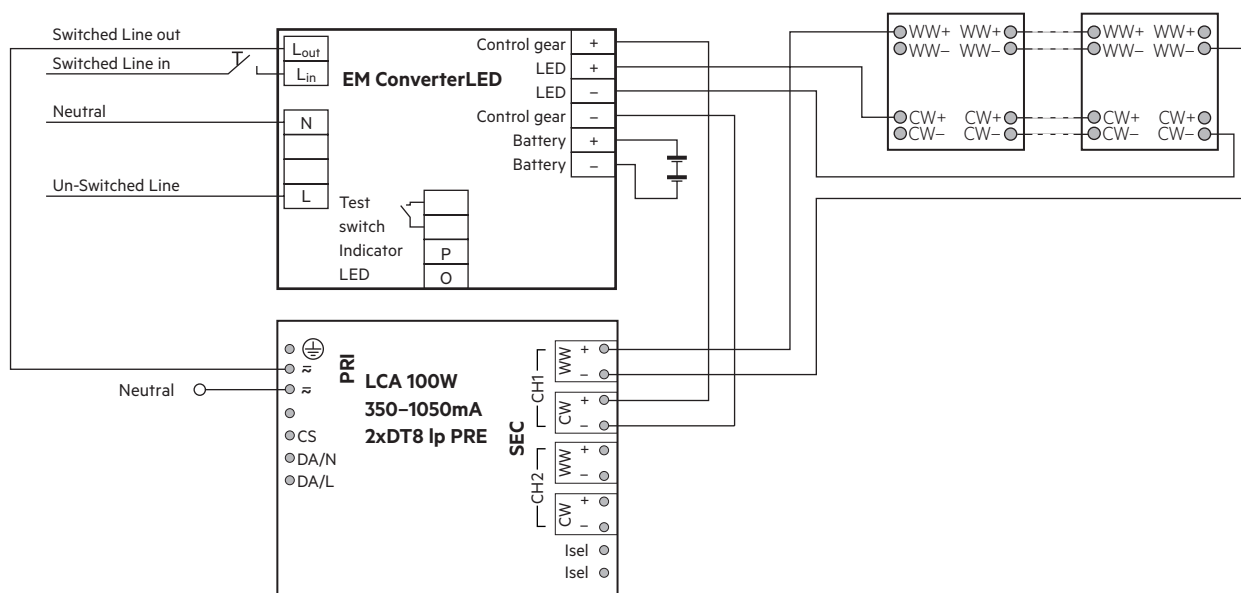
Verdrahtungsdiagramm für Notlicht
